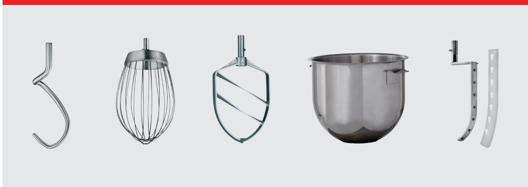
Крюк, венчик, Лопатка, скребок и дежа объемом 10 л из нержавеющей стали. Скребок с лезвием из нейлона или тефлона.
